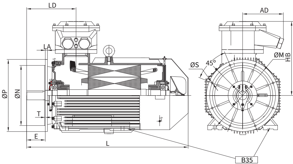
底脚及外形尺寸示意图
